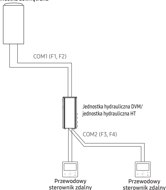
Jednostka zewnętrzna
